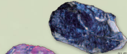
銅藍
