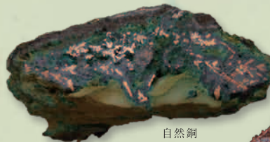
自然銅
