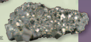
方鉛鉱
