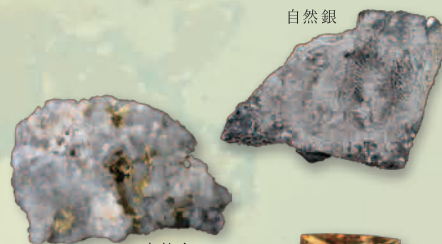
自然金
