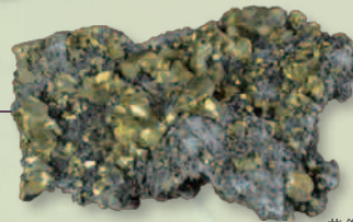
黄銅鉱
