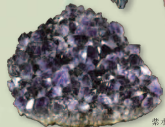
紫水晶
